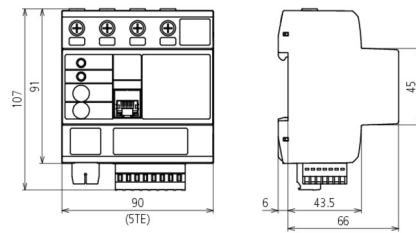
Maßbild DRC SD 1 1
