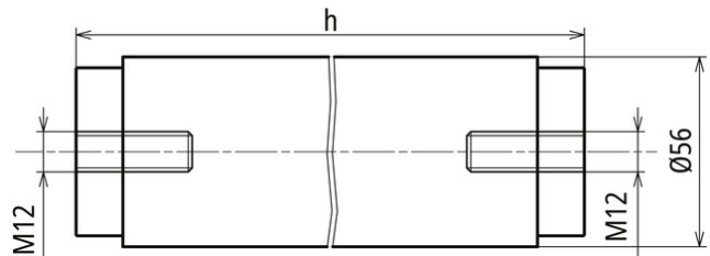
Maßbild SBKW 12/DH-I-0
