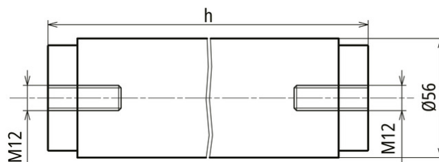
Maßbild SBKW 45/DH-I-0
