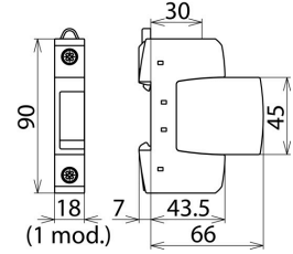
Dimension drawing DG SU 1P 240
