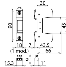
Dimension drawing DG SU 1P 347 R
