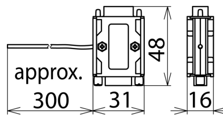
Dimension drawing FS 9E PB 6
