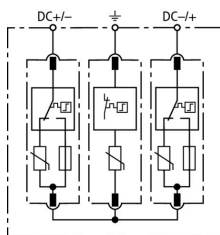
Schéma de principe du circuit DG M YPV SCI 1200
