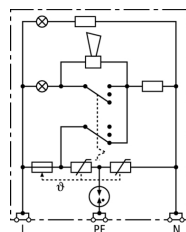
Schéma de principe du circuit DSA 230 LA
