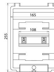
Dimensions IGA 6 IP54
