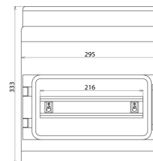
Dimensions IGA 12 IP54
