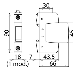
Dimensions DG S 275
