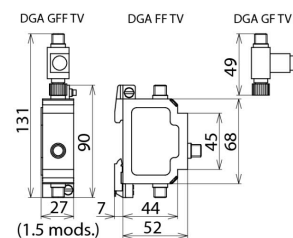
Dimensions DGA FF TV
