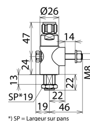
Dimensions DGA AG N
