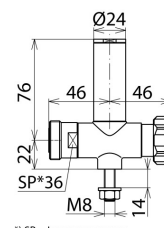
Dimensions DGA L4 7 16 S
