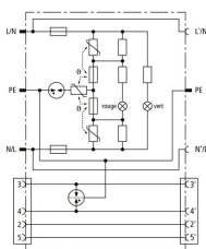
Schéma de principe du circuit DPRO 230 NT
