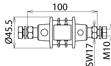
Dimensions EXFS 100
