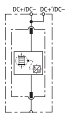
Schéma de principe du circuit DSE M 1 242
