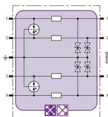
Schéma de principe du circuit BXT ML4 BE 36
