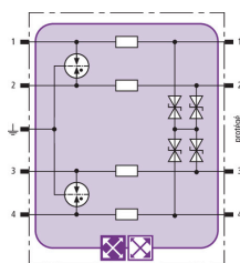
Schéma de principe du circuit BXT ML4 BC 24
