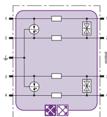
Schéma de principe du circuit BXT ML4 BD HF 24
