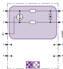
Schéma de principe du circuit BXT ML2 BD 180
