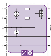
Schéma de principe du circuit BXT ML2 BE HFS 5
