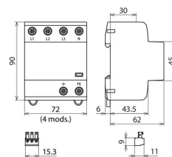
Dimensions DSH TNS 255 FM
