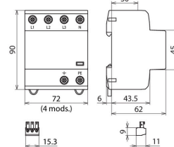
Dimensions DSH B TNS 255 FM
