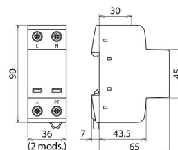
Dimensions DSH TN 255
