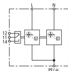
Schéma de principe du circuit DSH B TN 255 FM
