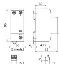
Dimensions DSH B TN 255 FM
