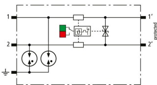
Circuit du BCO CL2 BD 48
