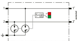
Schéma de principe BCO ML2 B 180
