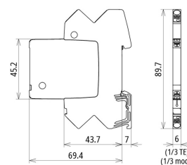
Dimension du BCO ML2 BD 12
