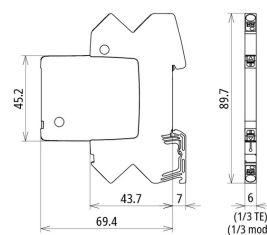
Dimension du BCO ML2 BD 48
