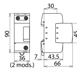
Dimensions DB M 1 320
