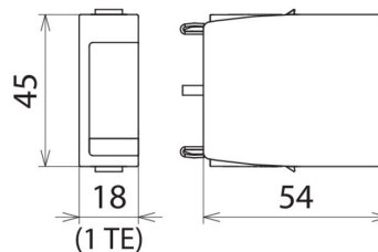
Dimensions DG MOD ACI 385
