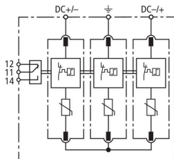
Schéma de principe du circuit DG M YPV 1200 FM - old
