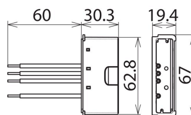
Dimensions DCOR L 2P 275 SO LTG
