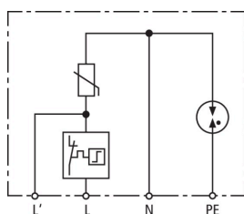
Schéma de principe du circuit DCOR L 2P 275 SO LTG
