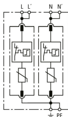
Schéma de principe du circuit DG MP TN 275
