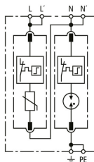
Schéma de principe du circuit DG MP TT 2P 275
