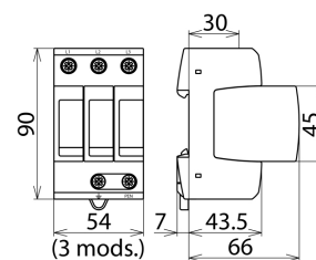
Dimensions DG M TNC 385
