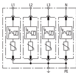
Schéma de principe du circuit DG M TNS 150
