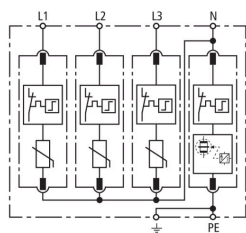
Schéma de principe du circuit DG M H TT 275
