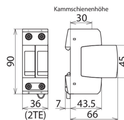
Dimensions DG M H TT 2P 275
