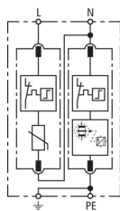
Schéma de principe du circuit DG M H TT 2P 275
