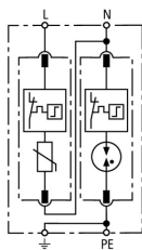
Schéma de principe du circuit DG M TT 2P 385
