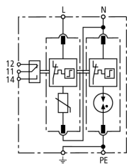
Schéma de principe du circuit DG M TT 2P 275 FM
