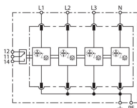
Schéma de principe du circuit DV M2 TNS 255 FM
