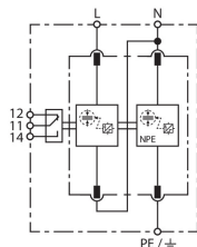
Schéma de principe du circuit DV M2 TT 2P 255 FM
