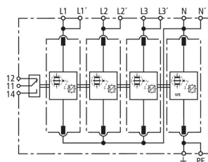
Schéma de principe du circuit DV M TT 255 FM
