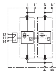
Schéma de principe du circuit DV M TN 255 FM
