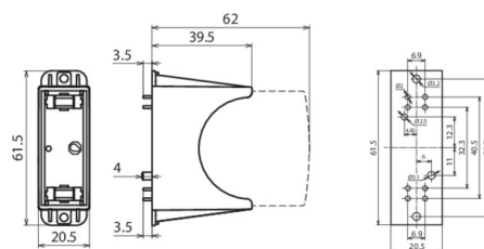
Dimensions DG PCB 385
