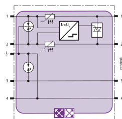
Schéma de principe du circuit BXTU ML2 BD S 0-180
