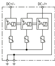
Schéma de principe du circuit DCU S 2 YPV 1+2 1200 2M 1S MC4
