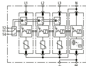
Schéma de principe du circuit DG M TT ACI 275 FM
